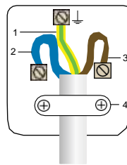
Voorbeeld van bedrading van stekker
