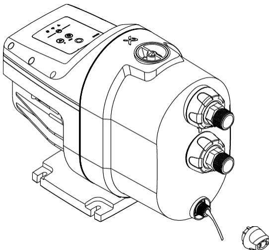
De pomp aftappen
