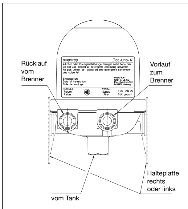
Ansicht Brennerseite
