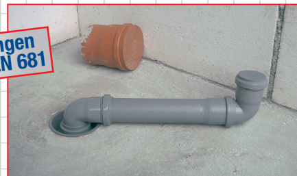
DN 200/160* Art. nr. 200160IR
