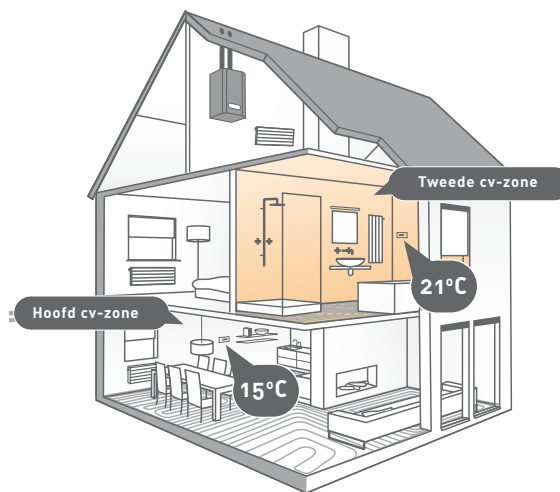
Woning met tweede cv-zone
